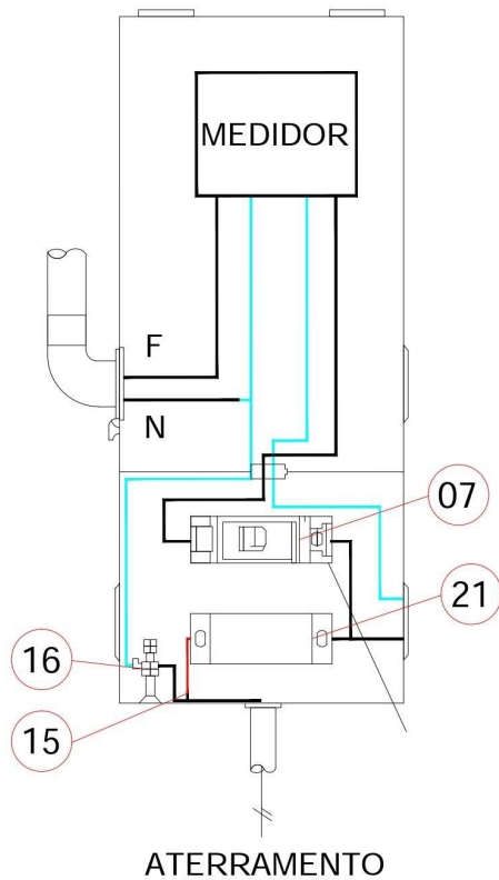
CAIXA DE MEDIÇÃO E PROTEÇÃO TIPO II PARA MEDIDOR MONOFÁSICO
