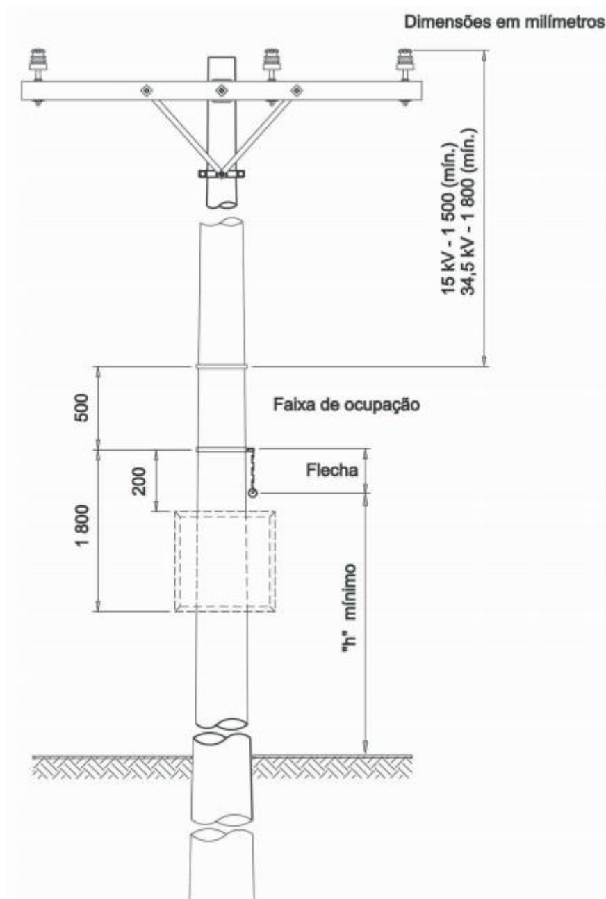
Figura A.3 — Afastamentos mínimos – Ocupação de poste com rede primária e sem
