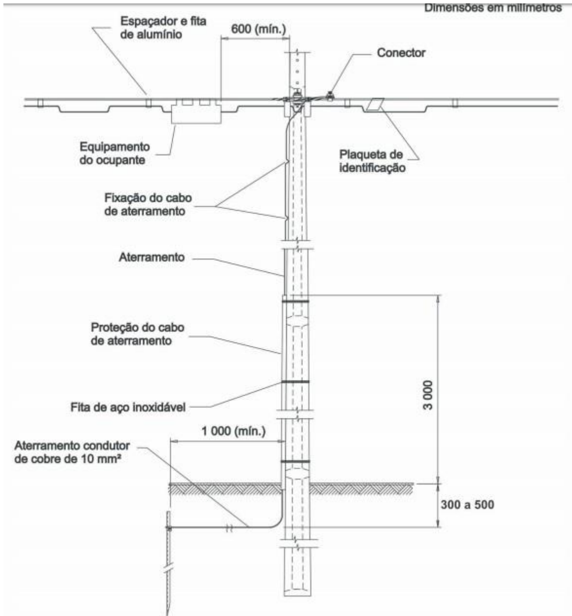
Figura A.9 — Espaçamentos mínimos e aterramento dos equipamentos do OCUPANTE nos postes
