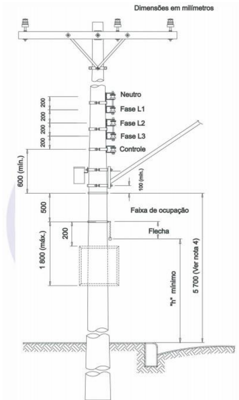
Figura A.2 — Afastamentos mínimos – Ocupação de poste com rede secundária
